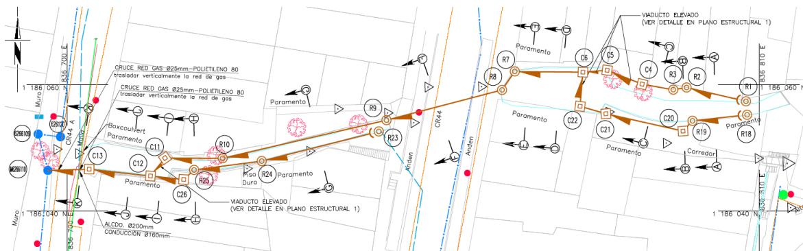
Esquema en planta de las obras proyectadas
